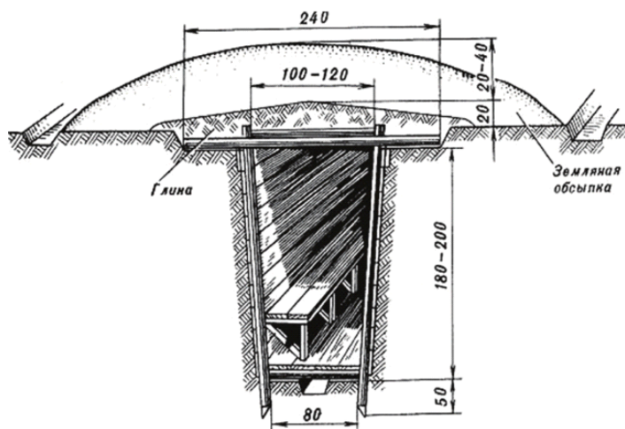
Рис. 6. Простейшие укрытия.
